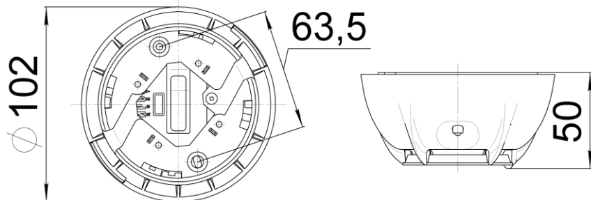
Рисунок 2 – Монтажная схема.
