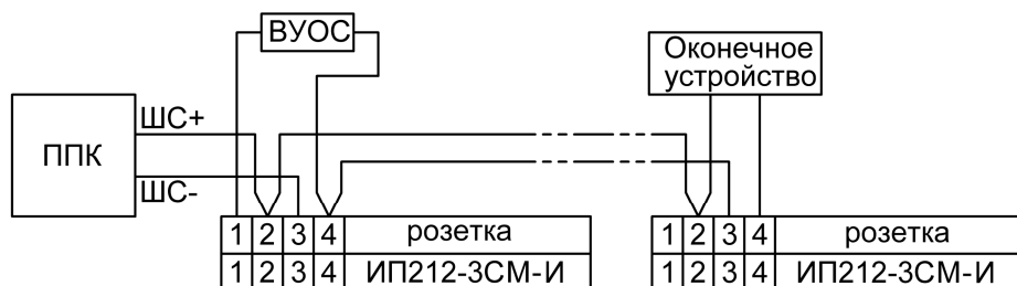
Рисунок 1 – Схема включения
