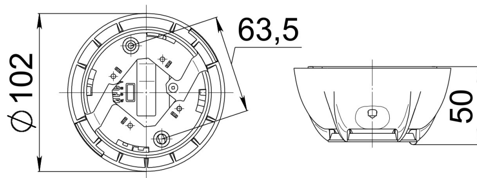
Рисунок 2 – Монтажная схема
